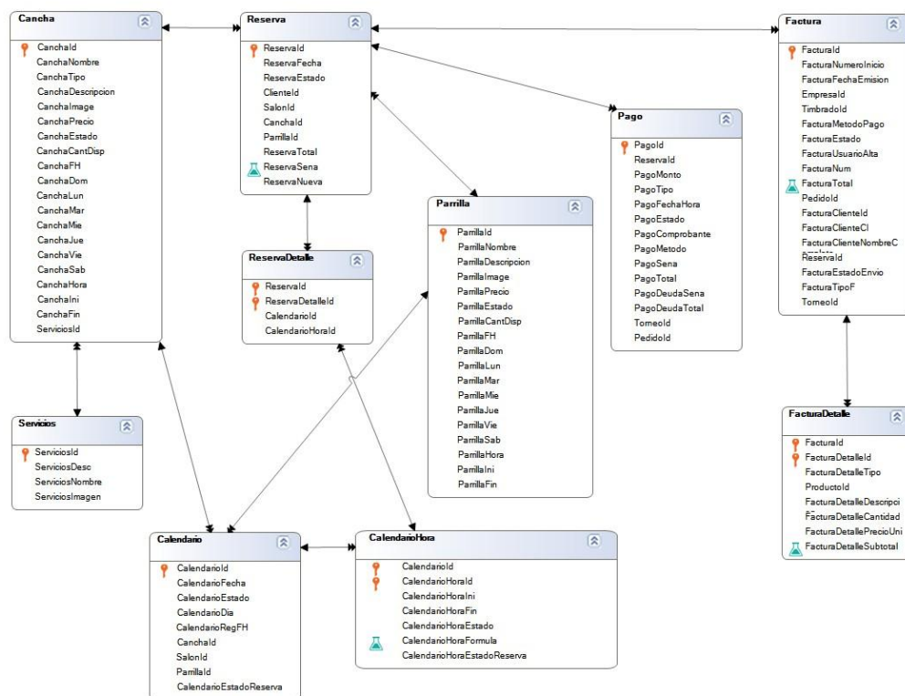
Diagrama ER Cancha
