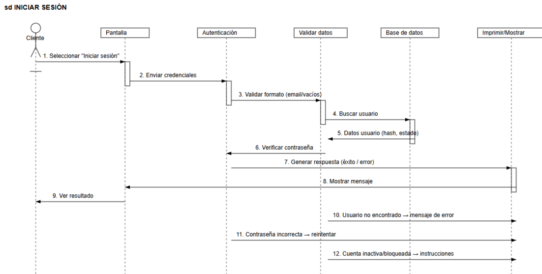
Figura 33. Diagrama de secuencia Inicio de Sesión
