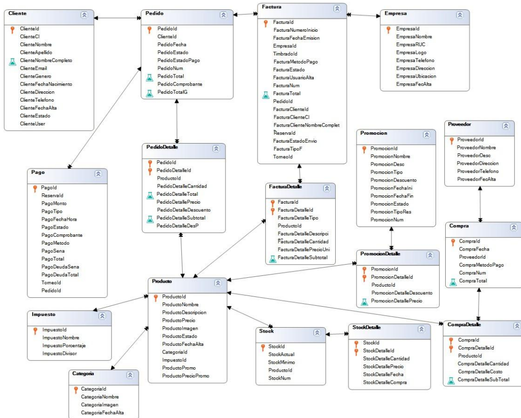
Diagrama ER Factura
